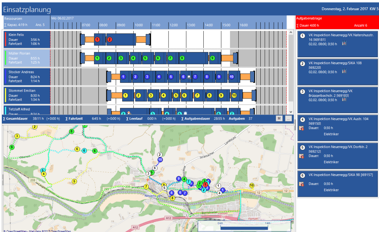
Abb.: Kartendarstellung der Aufgaben in der GS-Einsatzplanung
